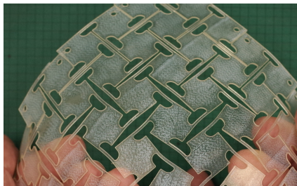
オーセティックな応答を示す2次元構造
