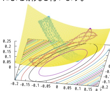
力学モデルのポテンシャル場とトラジェクトリー
