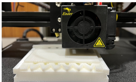
内部応力を埋め込んだ構造の3Dプリント
