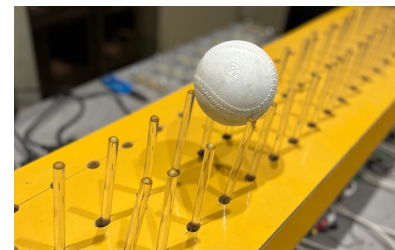
大自由度振動系により物体輸送
