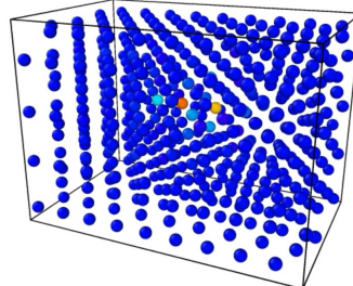
結晶内の非線形局在振動の分子動力学解析
